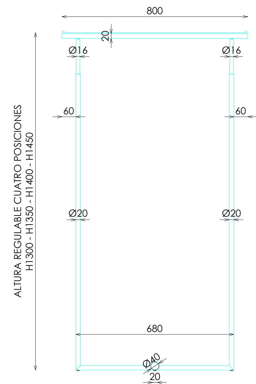
ALZADO
