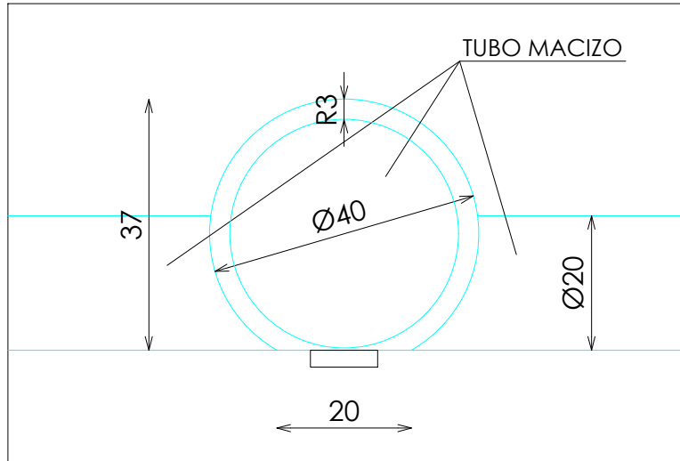
DETALLE BARRA CUELGUE
