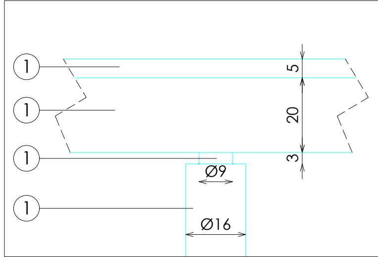
DETALLE B
