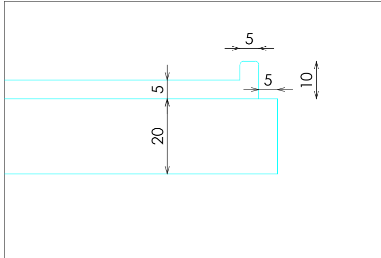
DETALLE C
