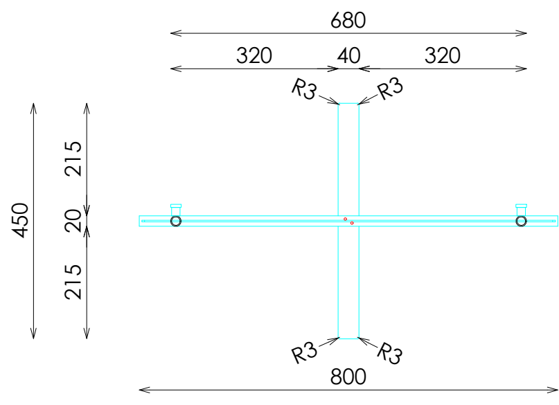
PLANTA
