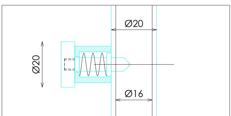
DETALLE SISTEMA ANCLAJE
