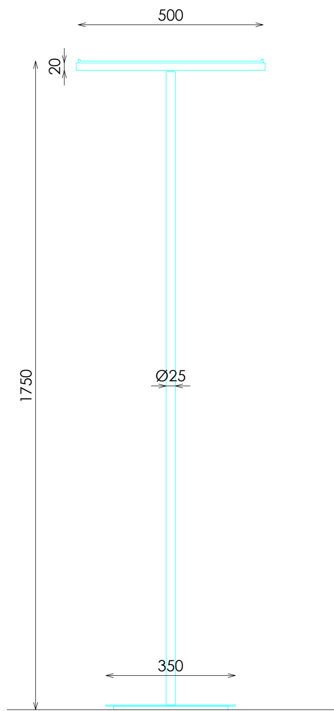
ALZADO
