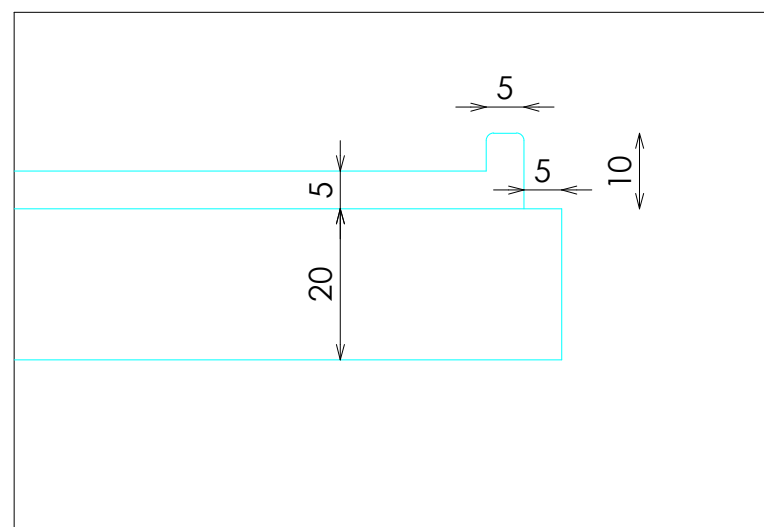
DETALLE B
