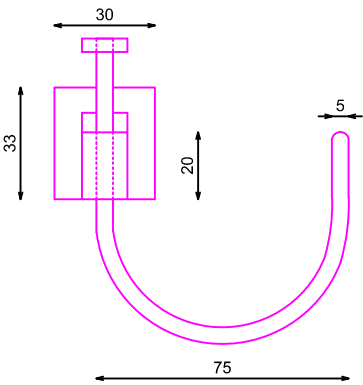
ALZADO
