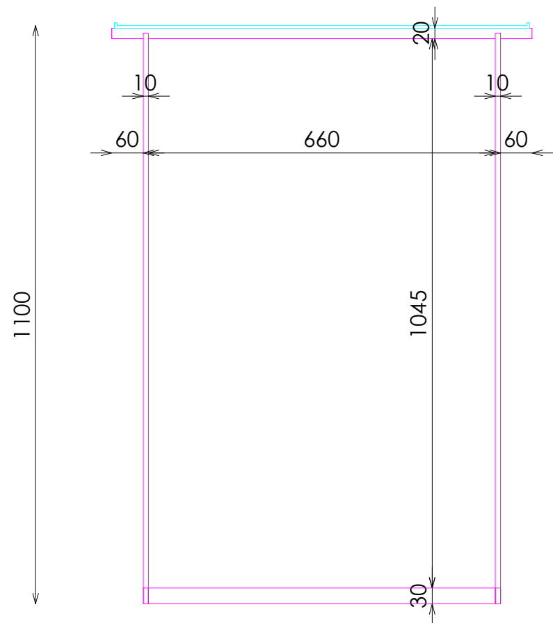
ALZADO
