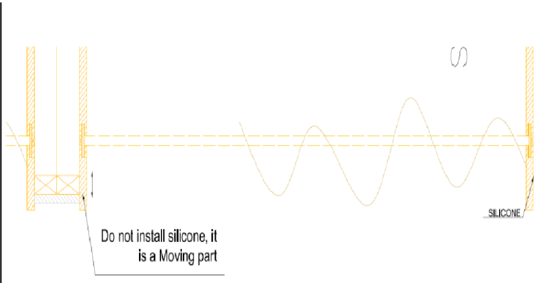
侧板安装示意图
