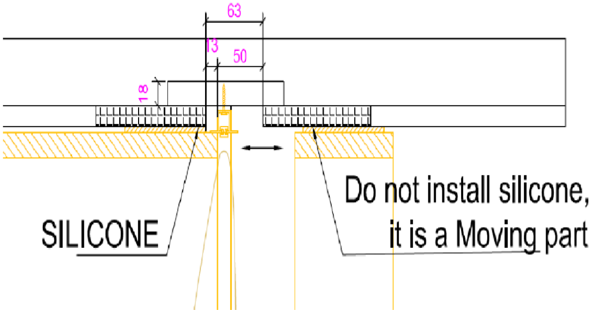
顶上布帘杆安装示意局部放大图
