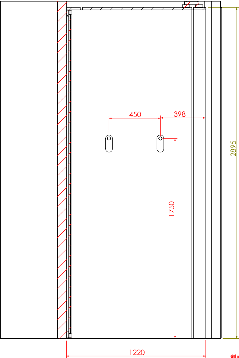
剖面 AI-AI
