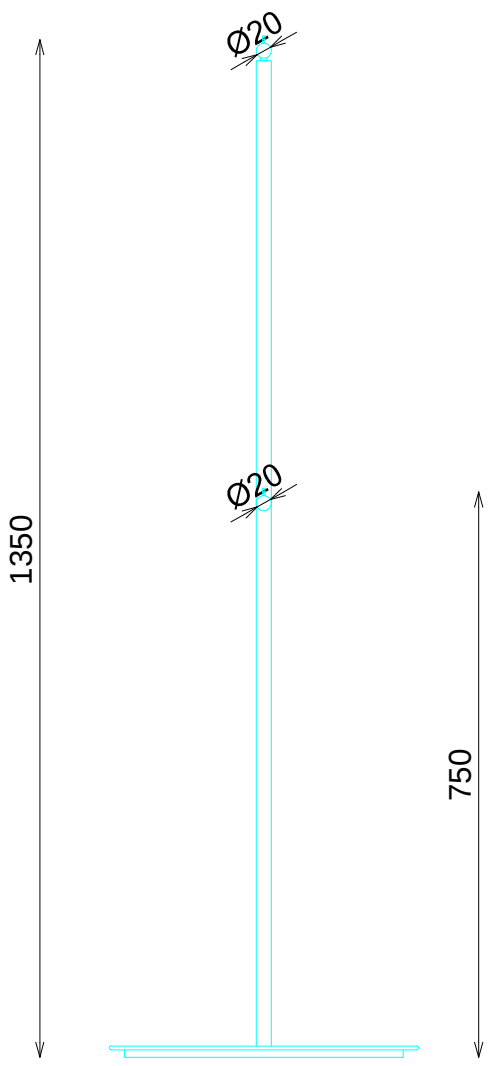
PERFIL
