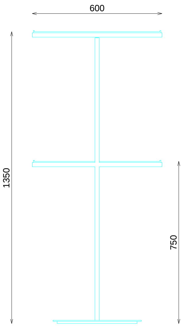
ALZADO
