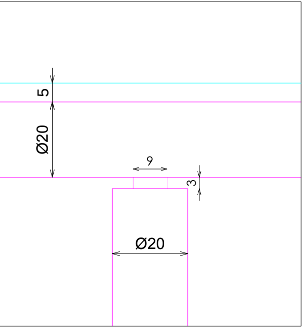
DETALLE C
