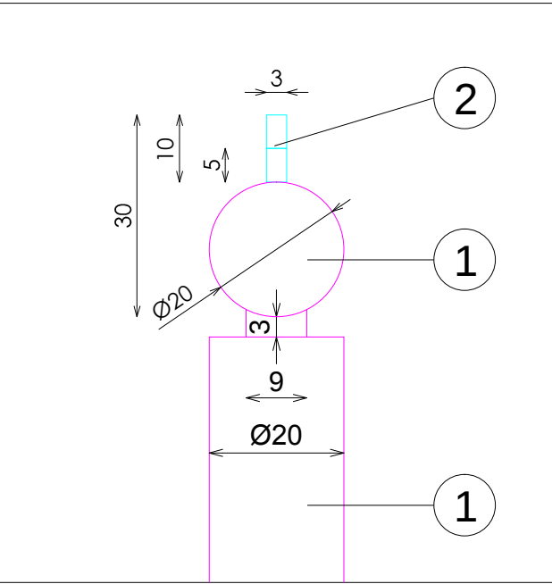
DETALLE ANTIROCE
