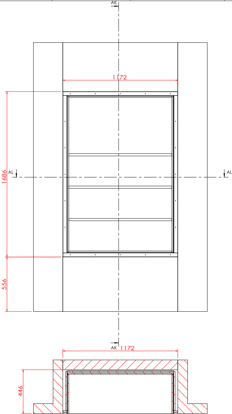
剖面 AL-AL
