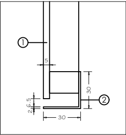
DETALLE DE MARCO ESPEJO
