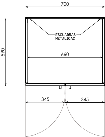
SECCIÓN PLANTA
