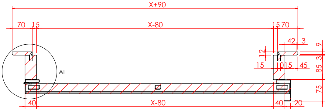
剖面 AG-AG 比例 1 : 8
