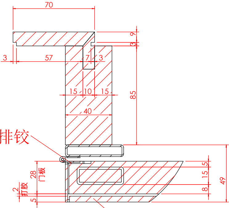
局部视图 AI 比例 1 : 2
