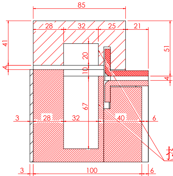
局部视图 AI 比例 1:2
