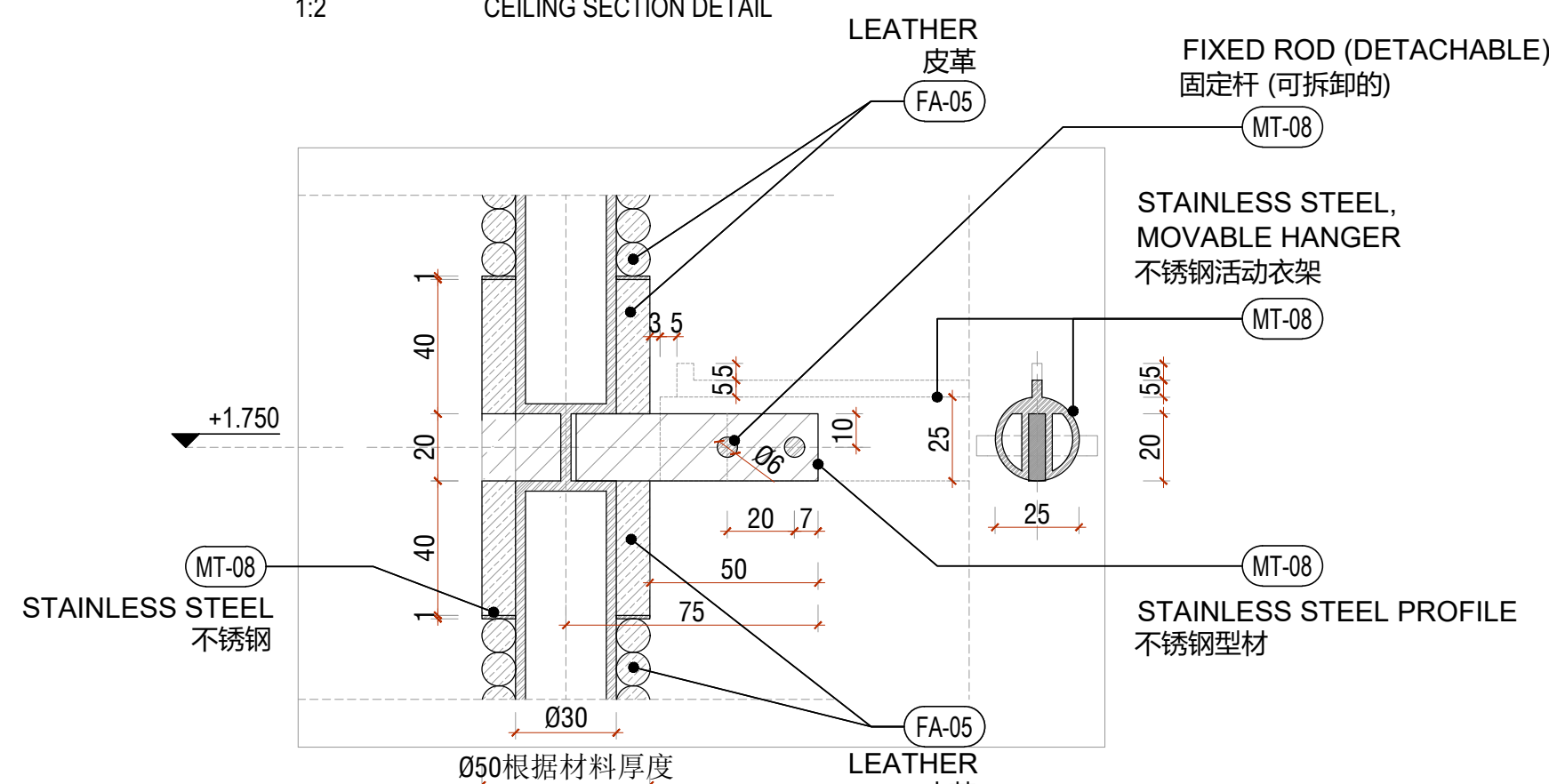
6 剖面节点 1:2 SECTION DETAIL
