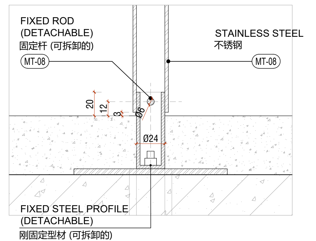
7 地面剖面节点 1:2 FLOOR SECTION DETAIL
