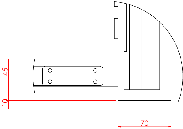
局部视图 AH 比例 1 : 3
