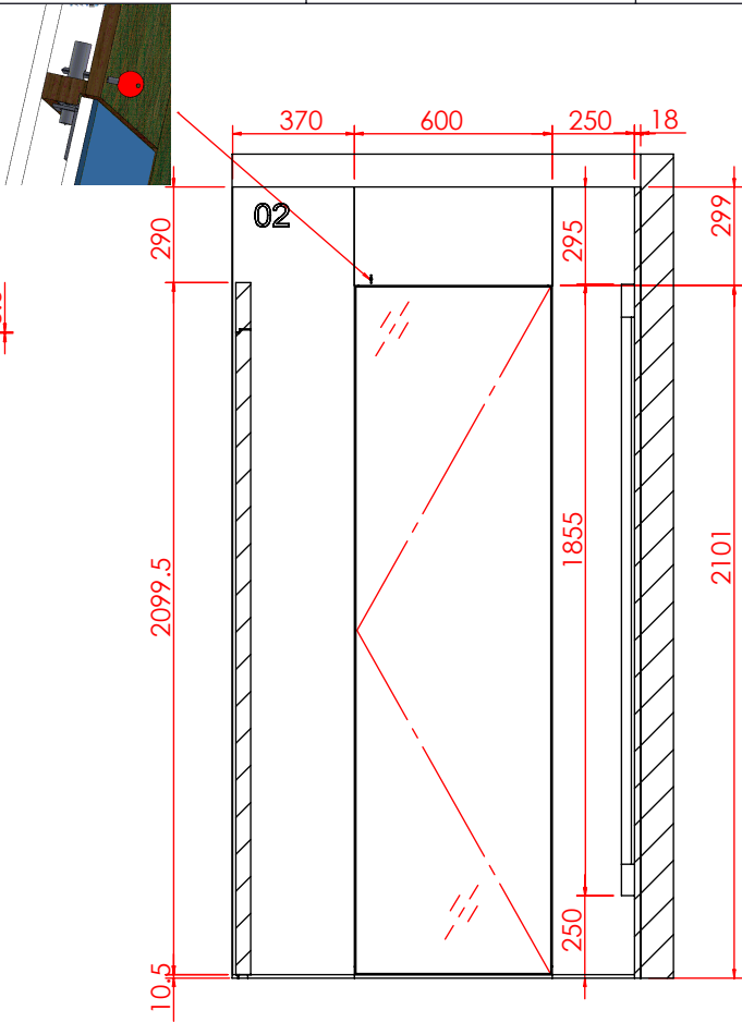
剖面 AJ-AJ
