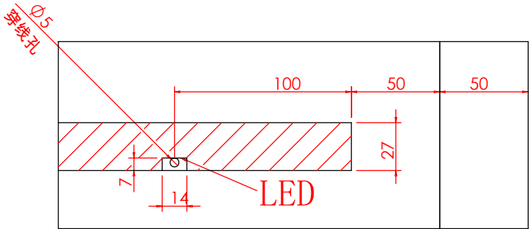
局部视图 AI 比例 1 : 3
