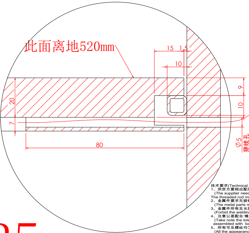
局部视图 AK 比例 1 : 1
