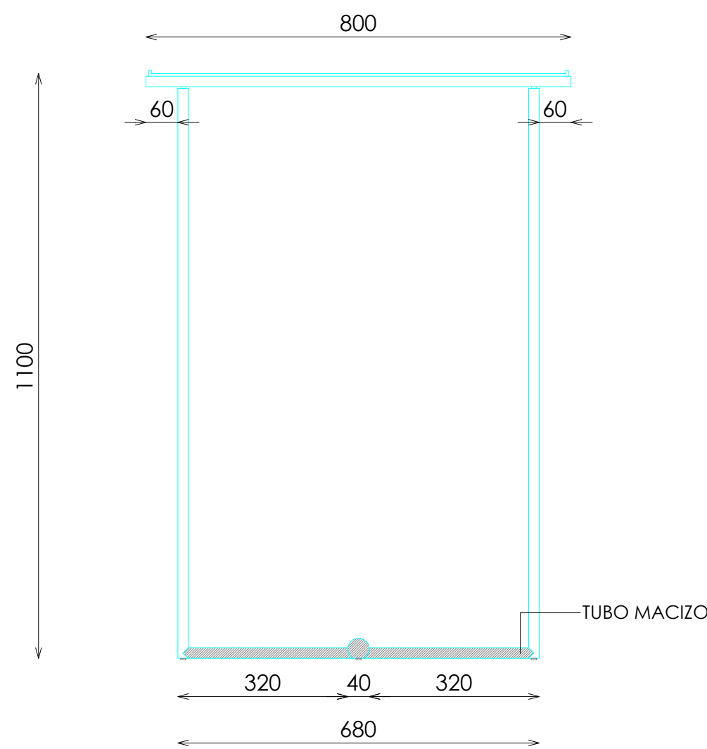
ESTRUCTURA
