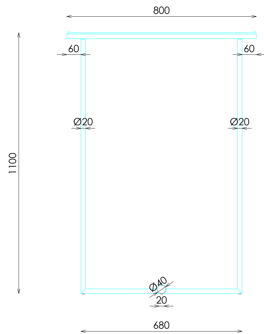
ALZADO
