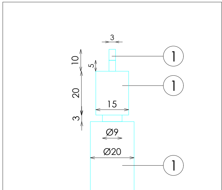
DETALLE BARRA CUELQUE
