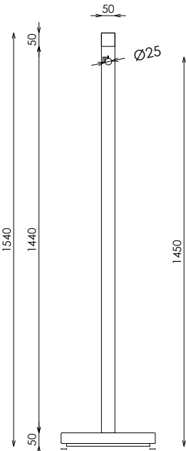
PERFIL SECCIONADO
