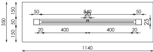
PLANTA SECCIONADA
