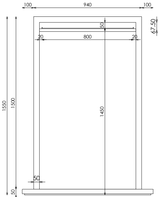
ALZADO
