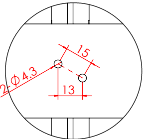
局部视图 AG 比例 1:2
