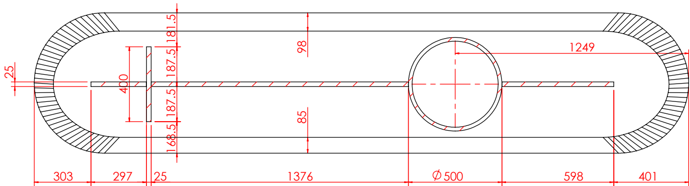
剖面 AG-AG
