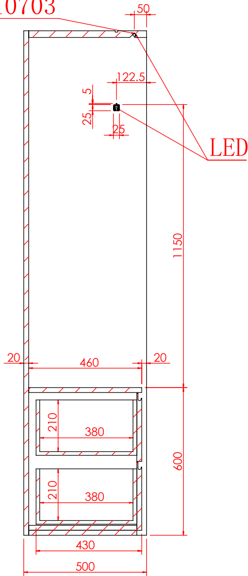
剖面 AG-AG
