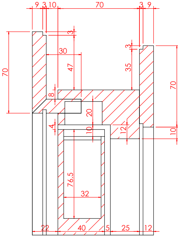
局部视图 AI 比例 1 : 2
