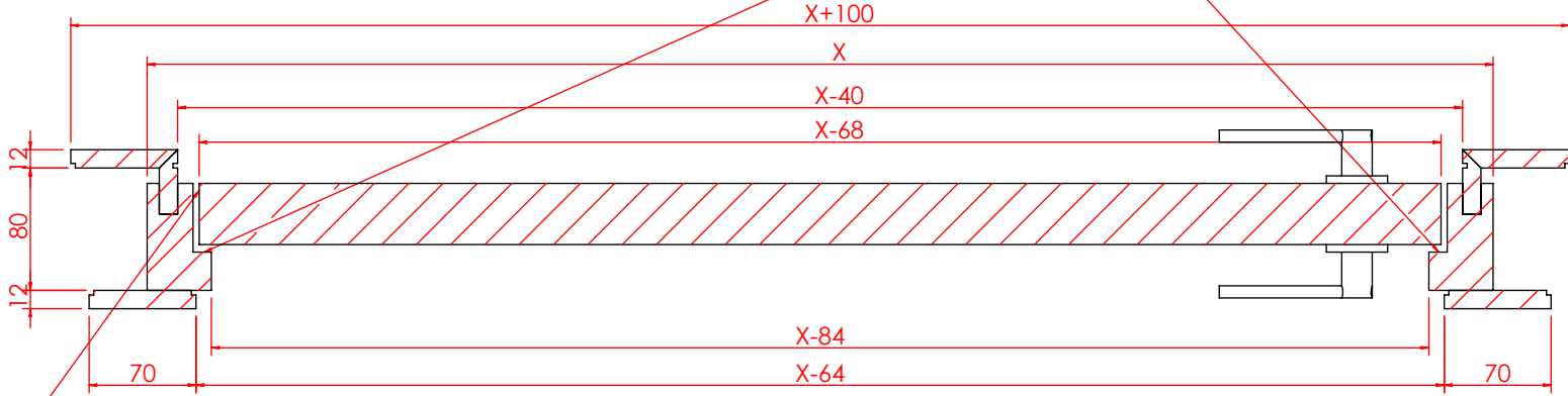
剖面 AG-AG 比例 1 : 5
