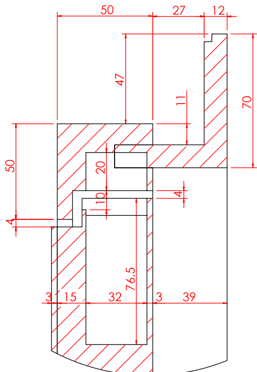
局部视图 AI 比例 1 : 2
