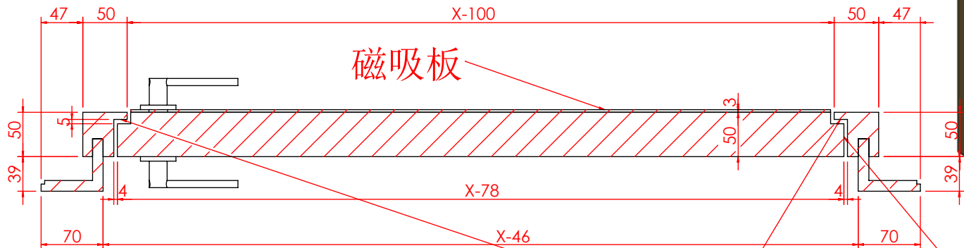
剖面 AG-AG 比例 1 : 6
