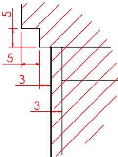
局部视图 AK 比例 1:1
