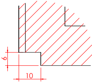
局部视图 AL 比例 1:1
