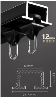
布帘杆参考款式
