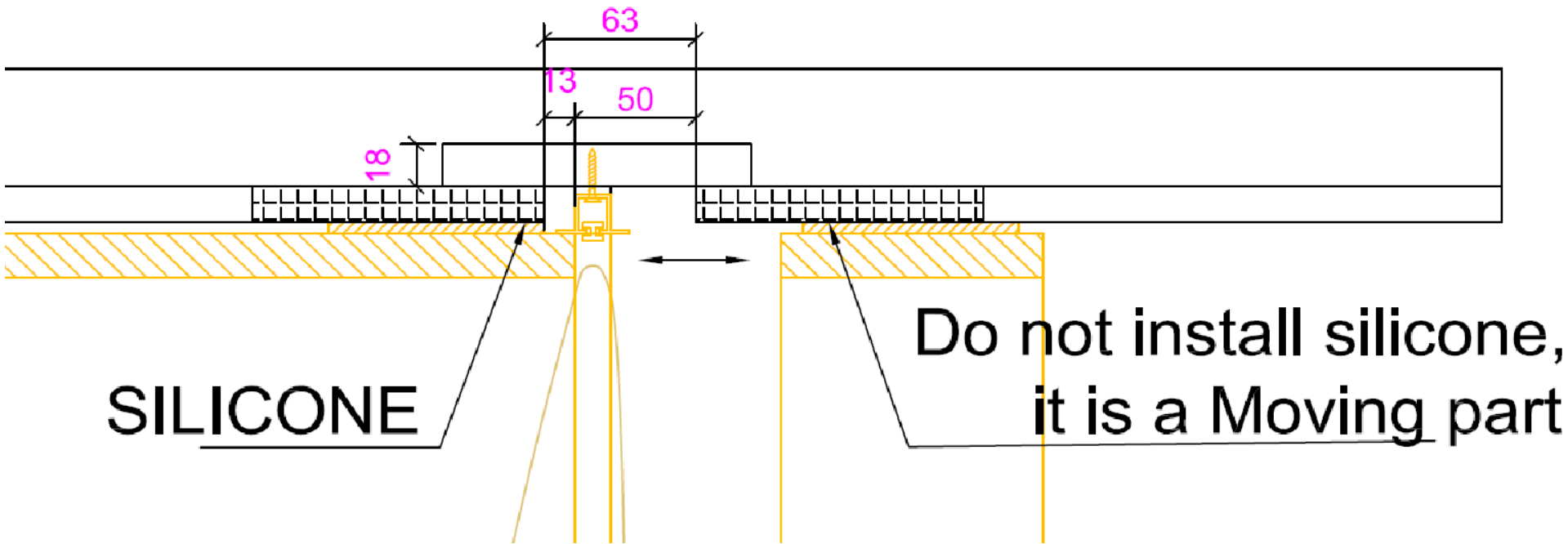
顶上布帘杆安装示意局部放大图
