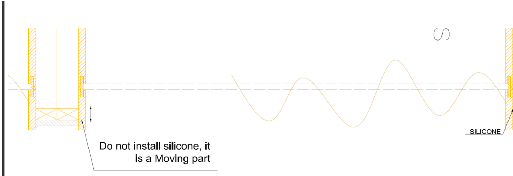
侧板安装示意图
