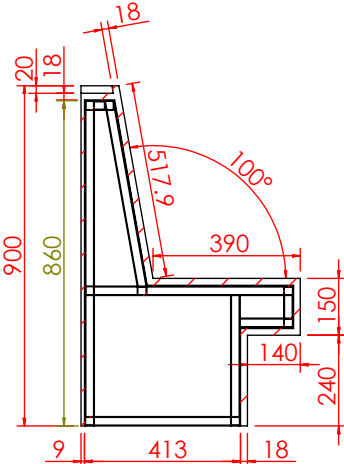
剖面 AJ-AJ
