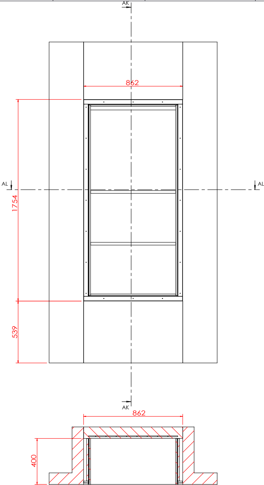
剖面 AL-AL
