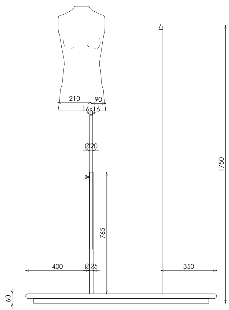
ALZADO FRONTAL
