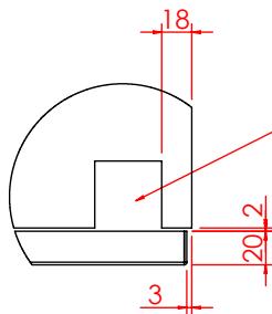
局部视图 AL 比例 1 : 5
