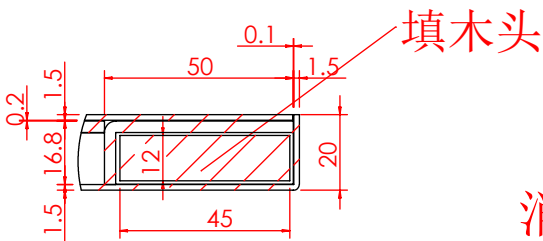
局部视图 AK 比例 1 : 2
