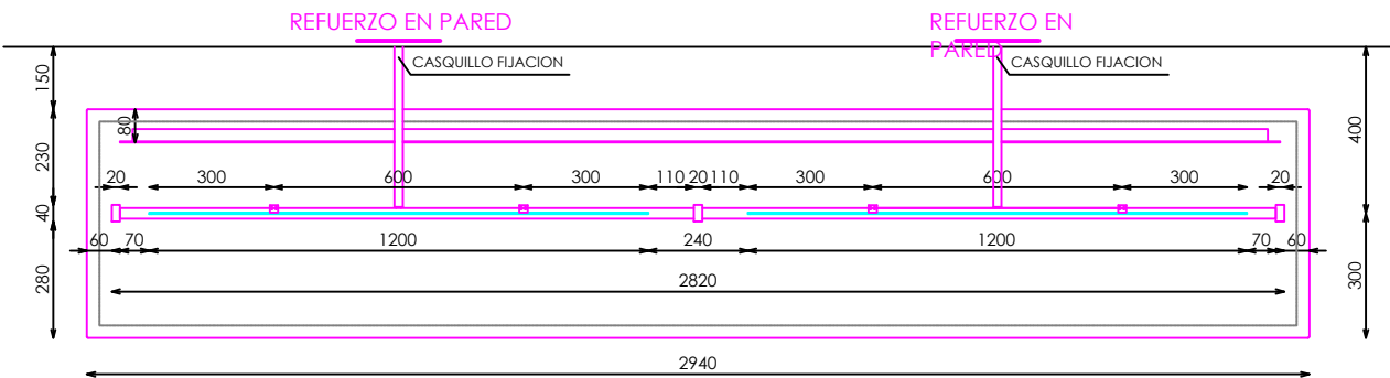
PLANTA
