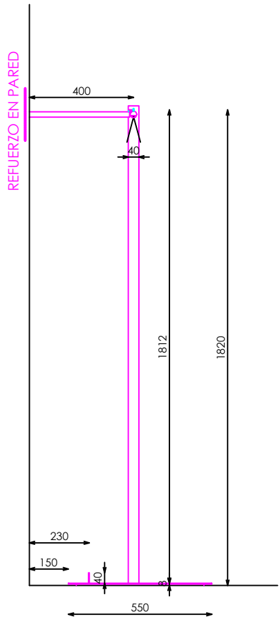
PERFIL SECCIONADO
