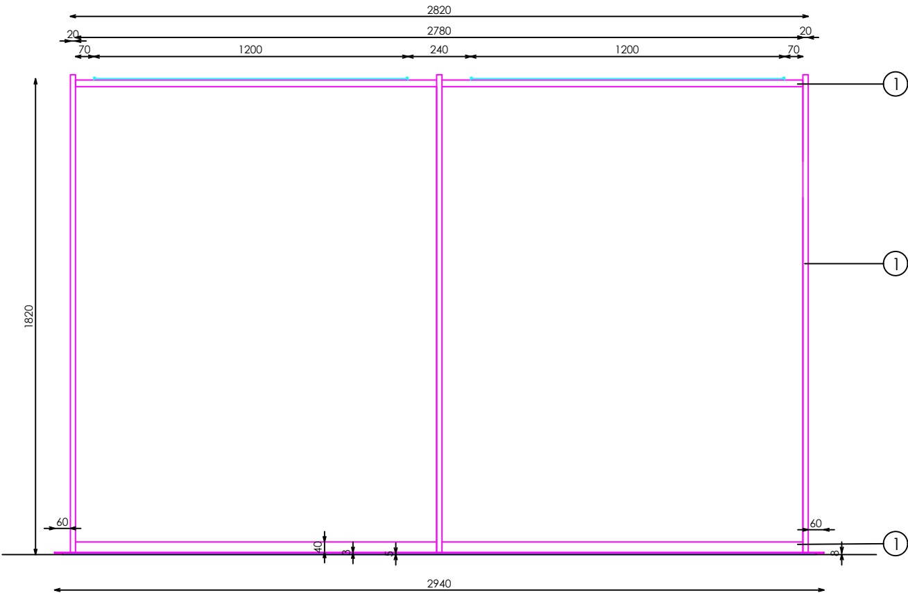
ALZADO SECCIONADO
