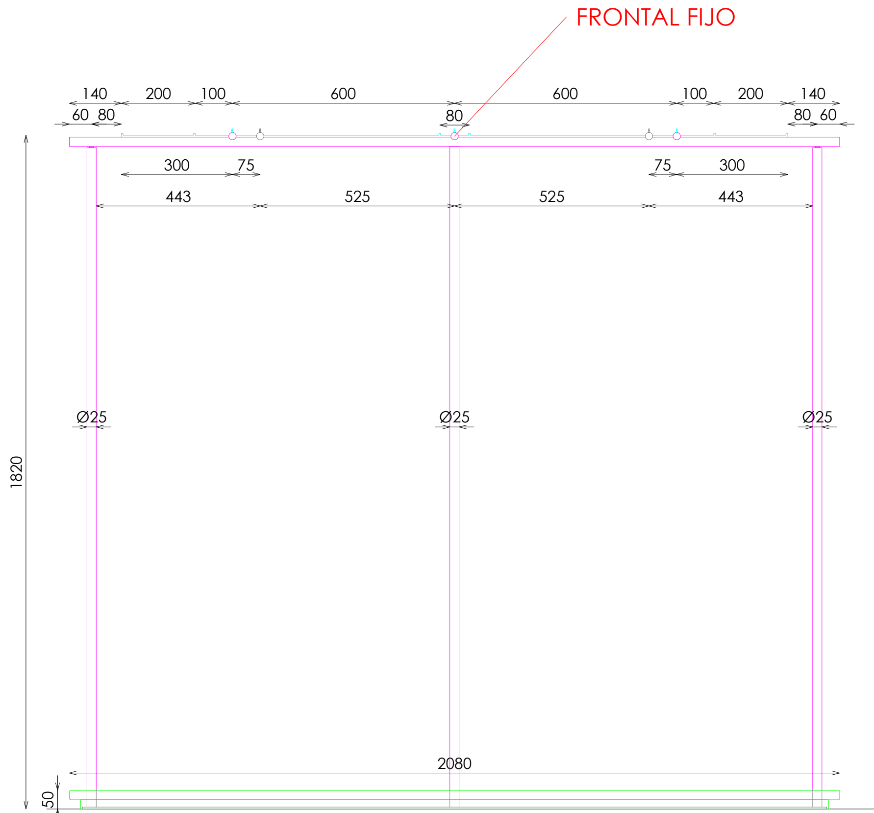
ALZADO FRONTAL
