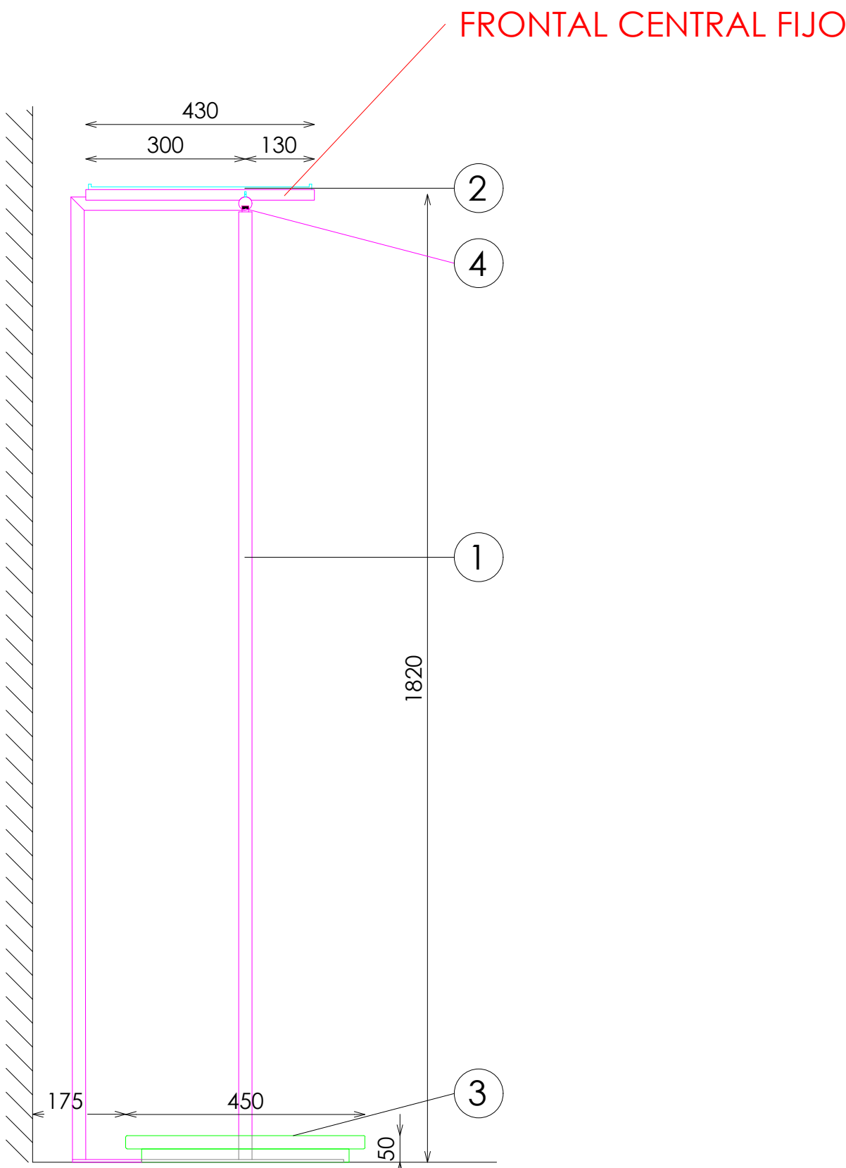
SECCIÓN
