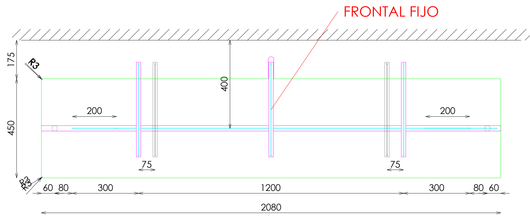
PLANTA
