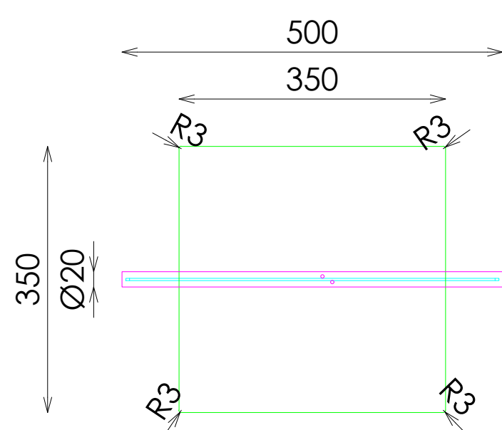
PLANTA
