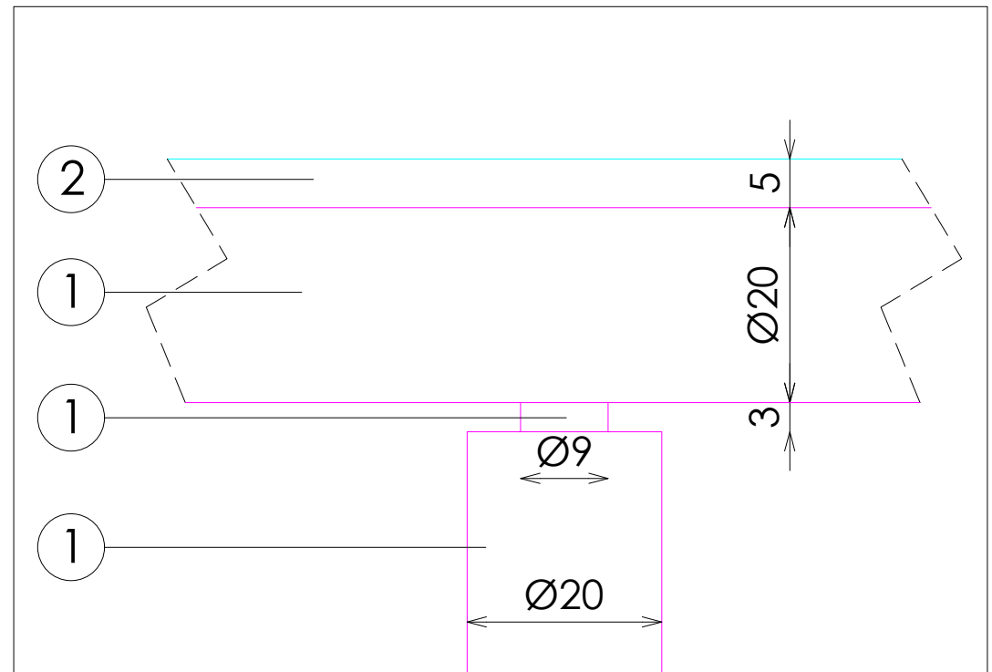
DETALLE B
