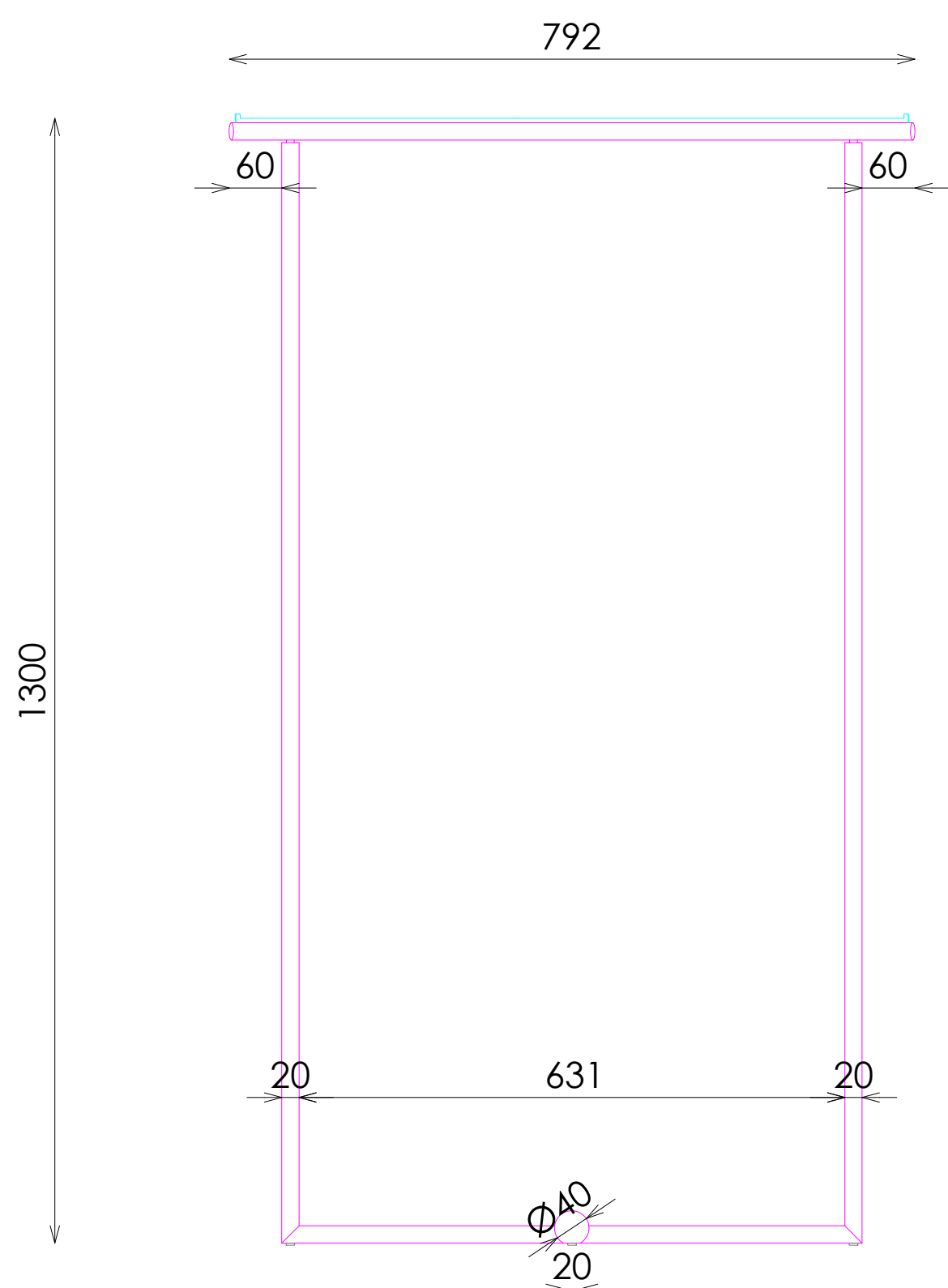
ALZADO
