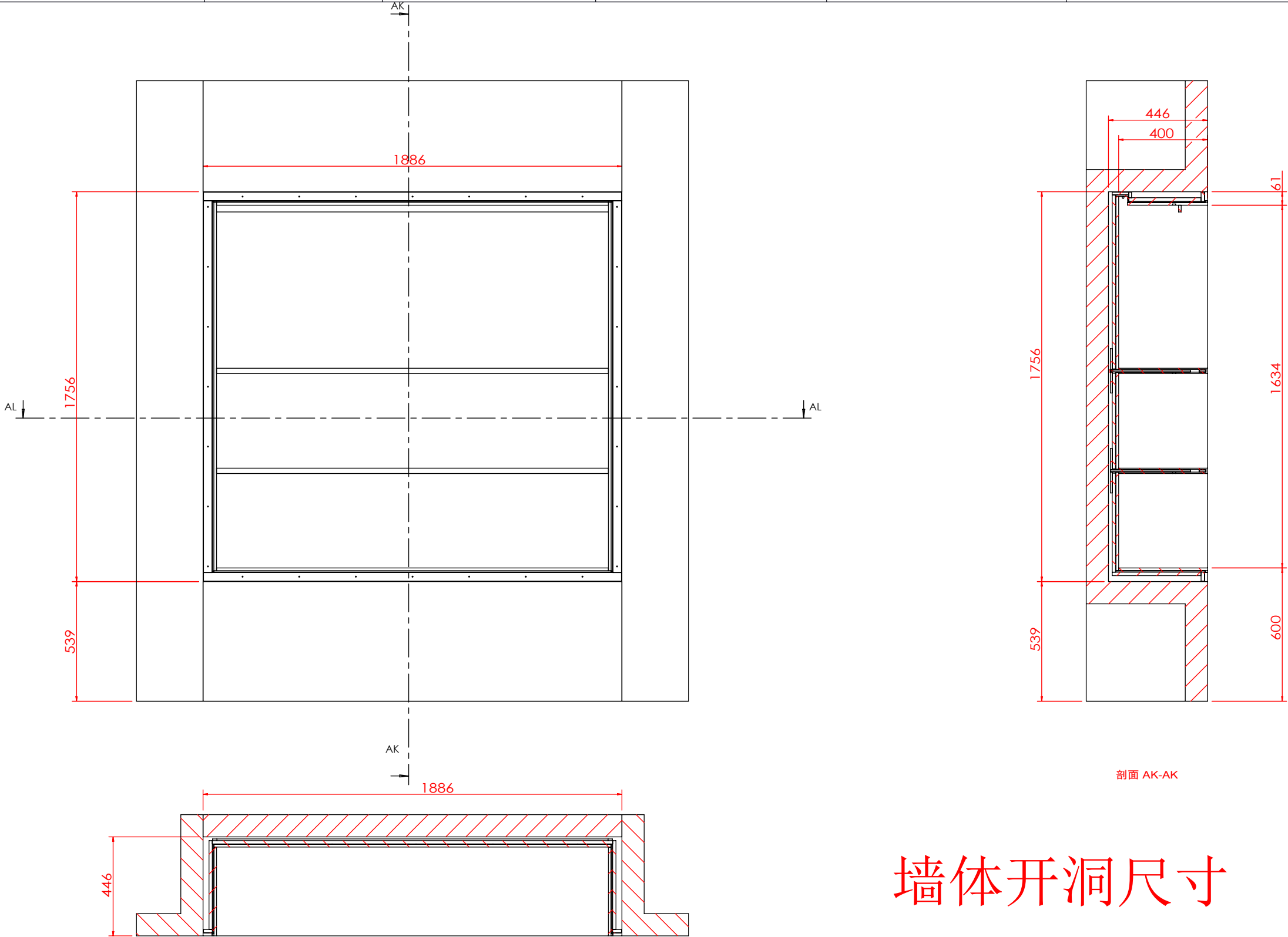
剖面 AL-AL
