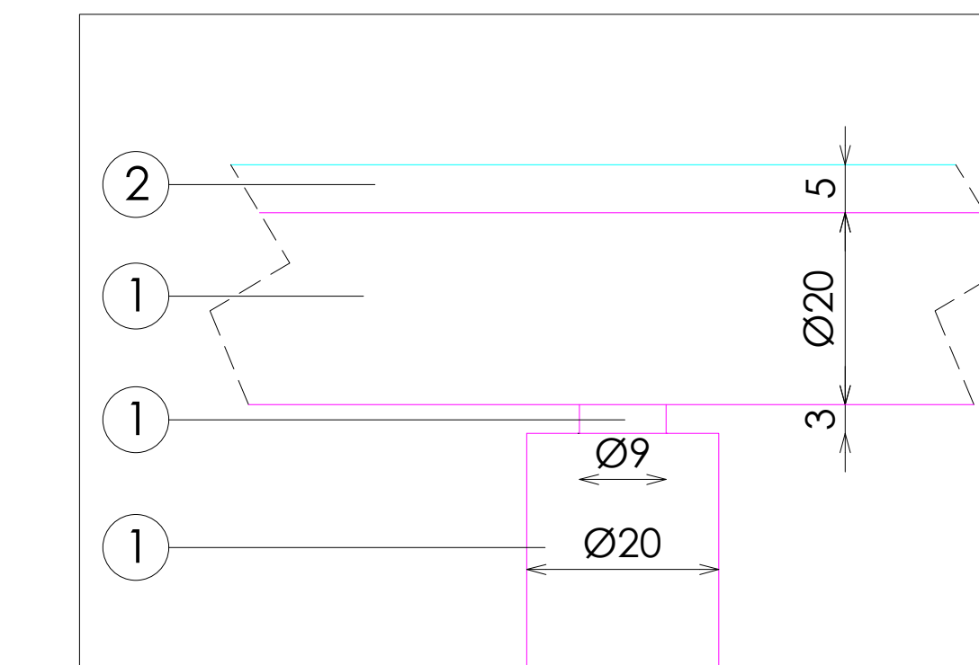
DETALLE B
