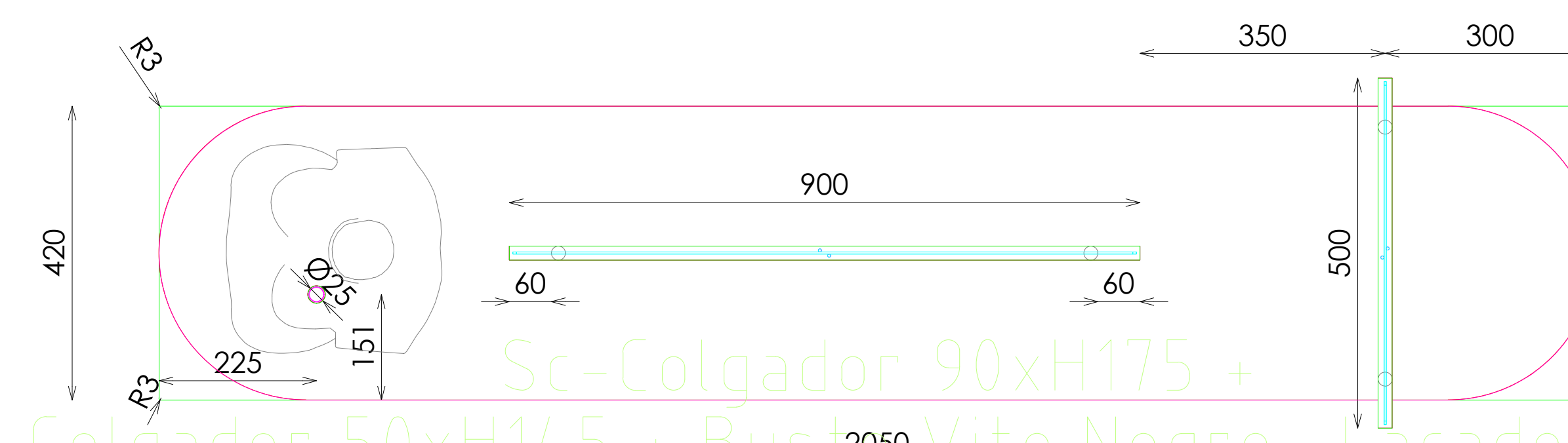
PLANTA
