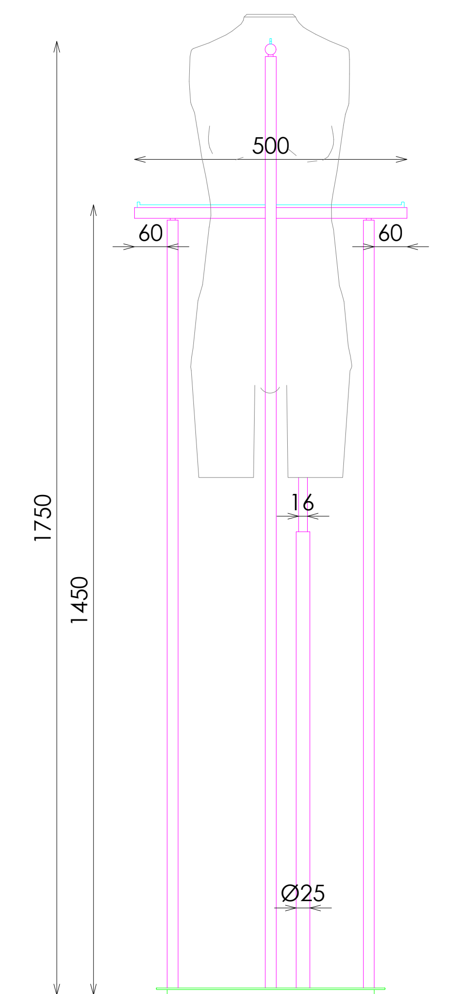
ALZADO FRONTAL
