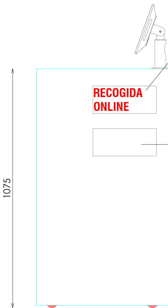
ALZADO LATERAL
