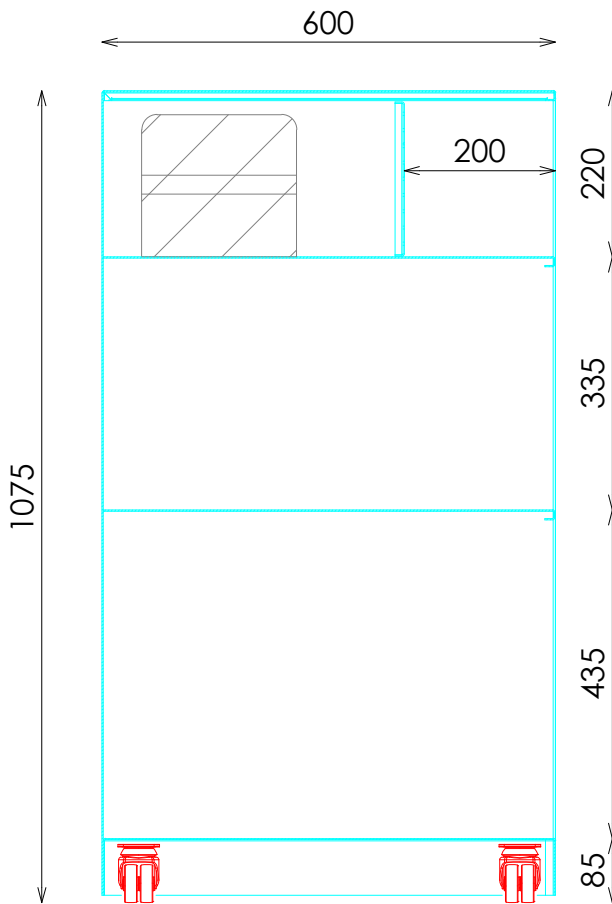
SECCIÓN
