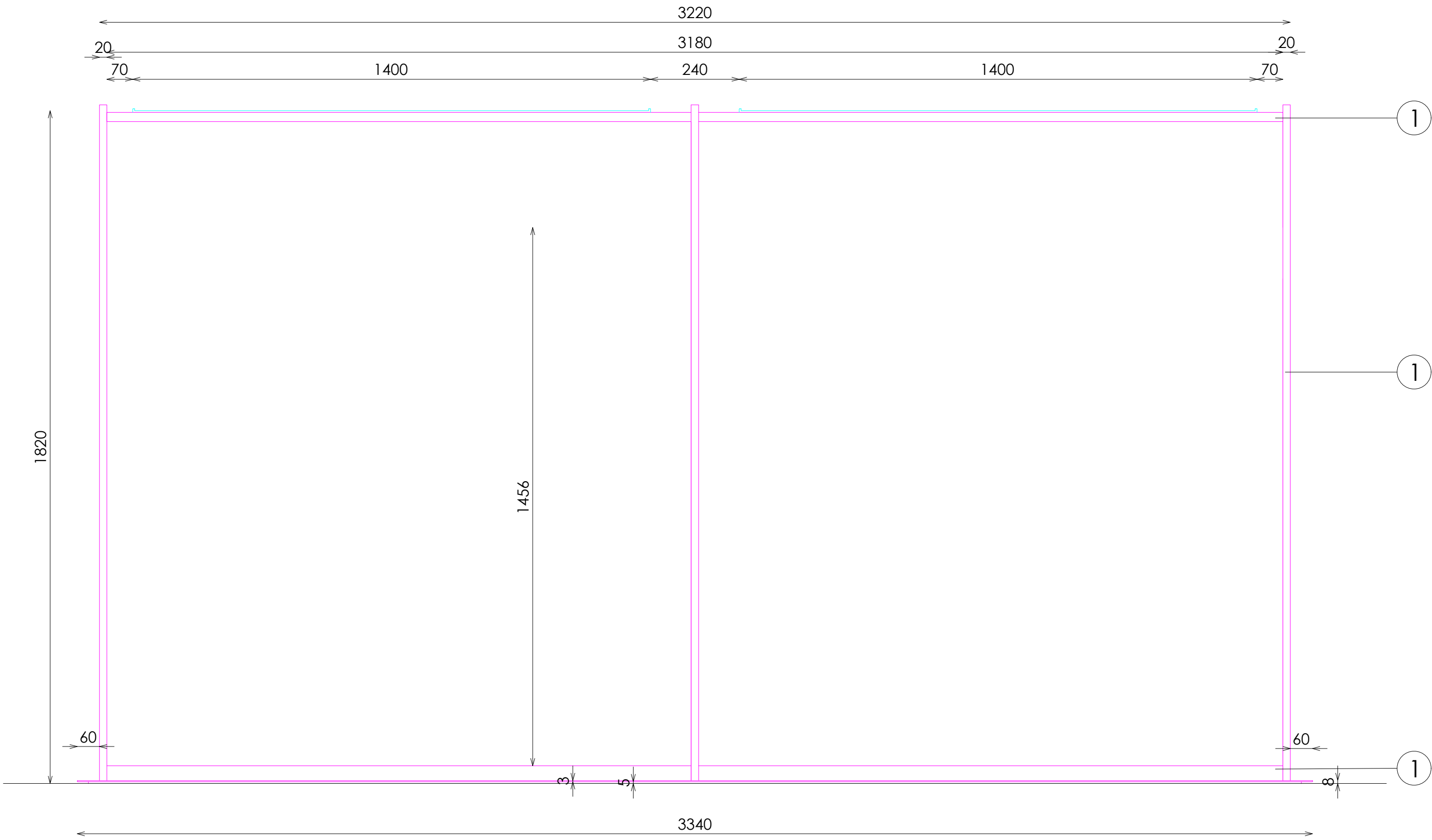
ALZADO SECCIONADO
