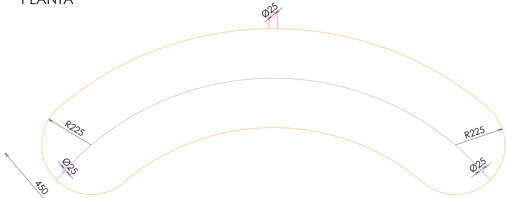
PLANTA
