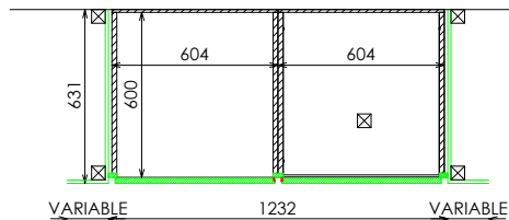
PLANTA 60-ST
