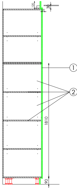
SECCION
