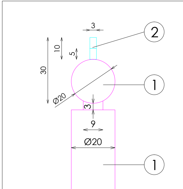
DETALLE ANTIROCE
