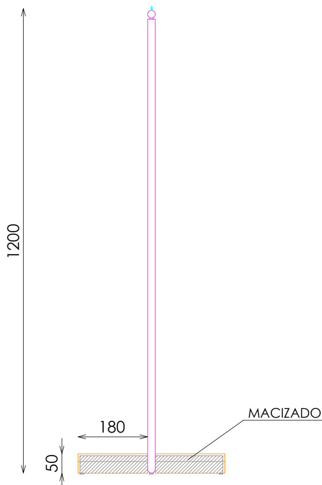
PERFIL
