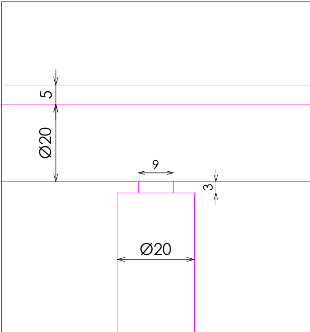
DETALLE C
