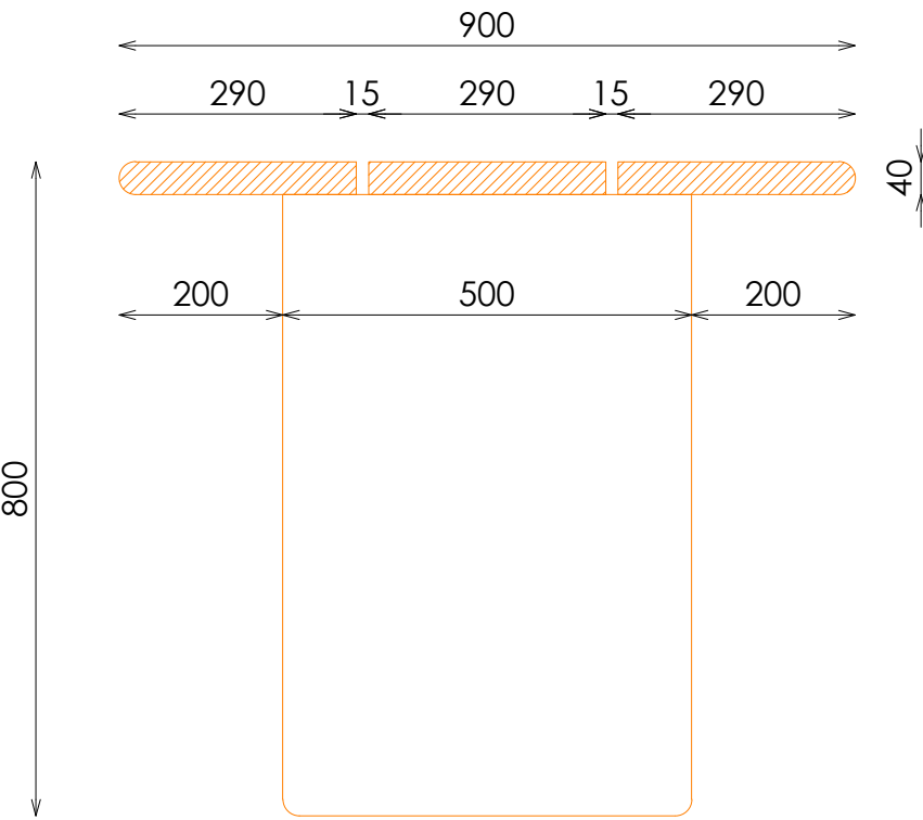
PERFIL
