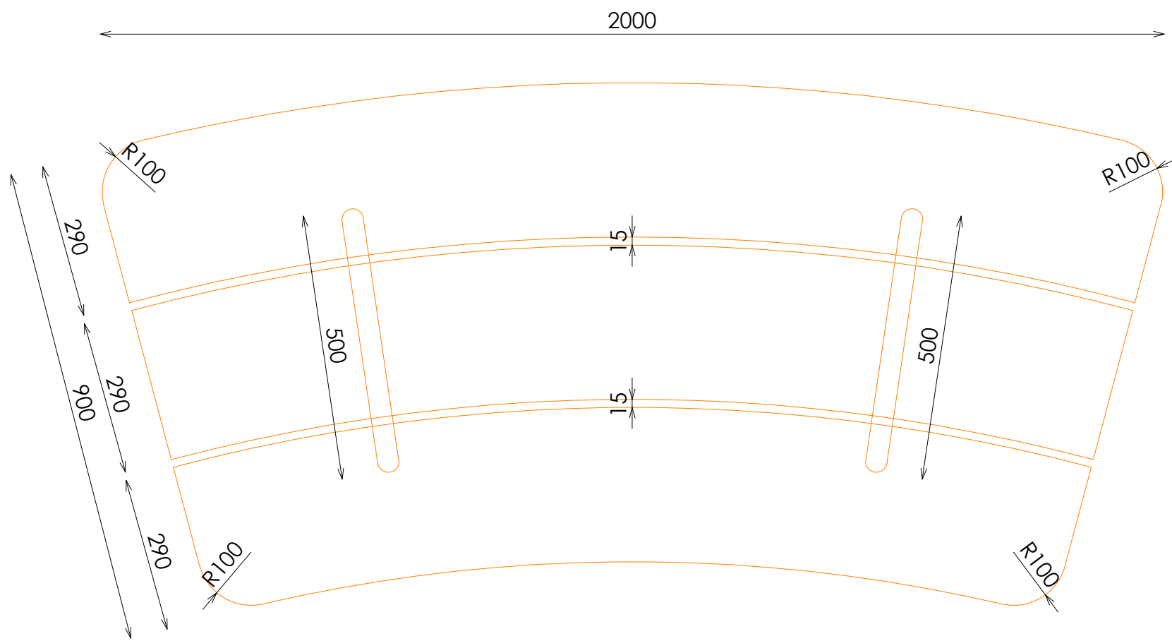
PLANTA
