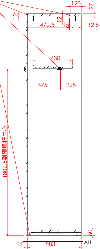
剖面 AG-AG
