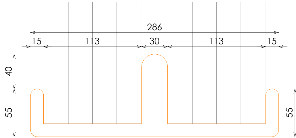
ALZADO
