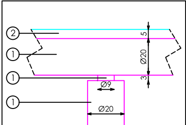
DETALLE B
