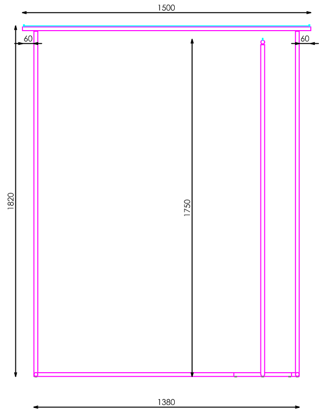
ALZADO
