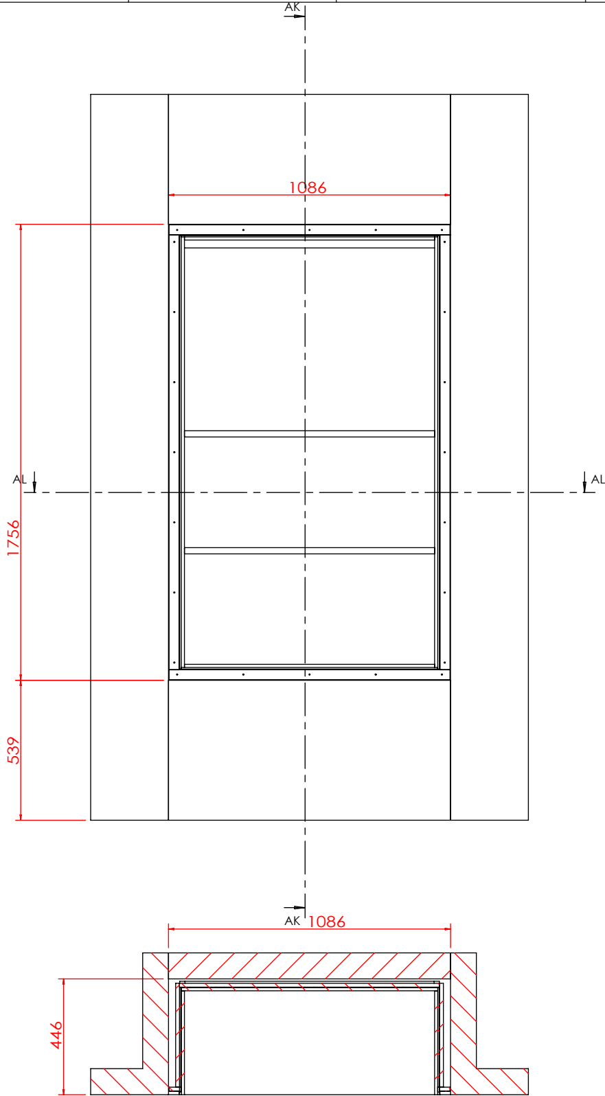
剖面 AL-AL
