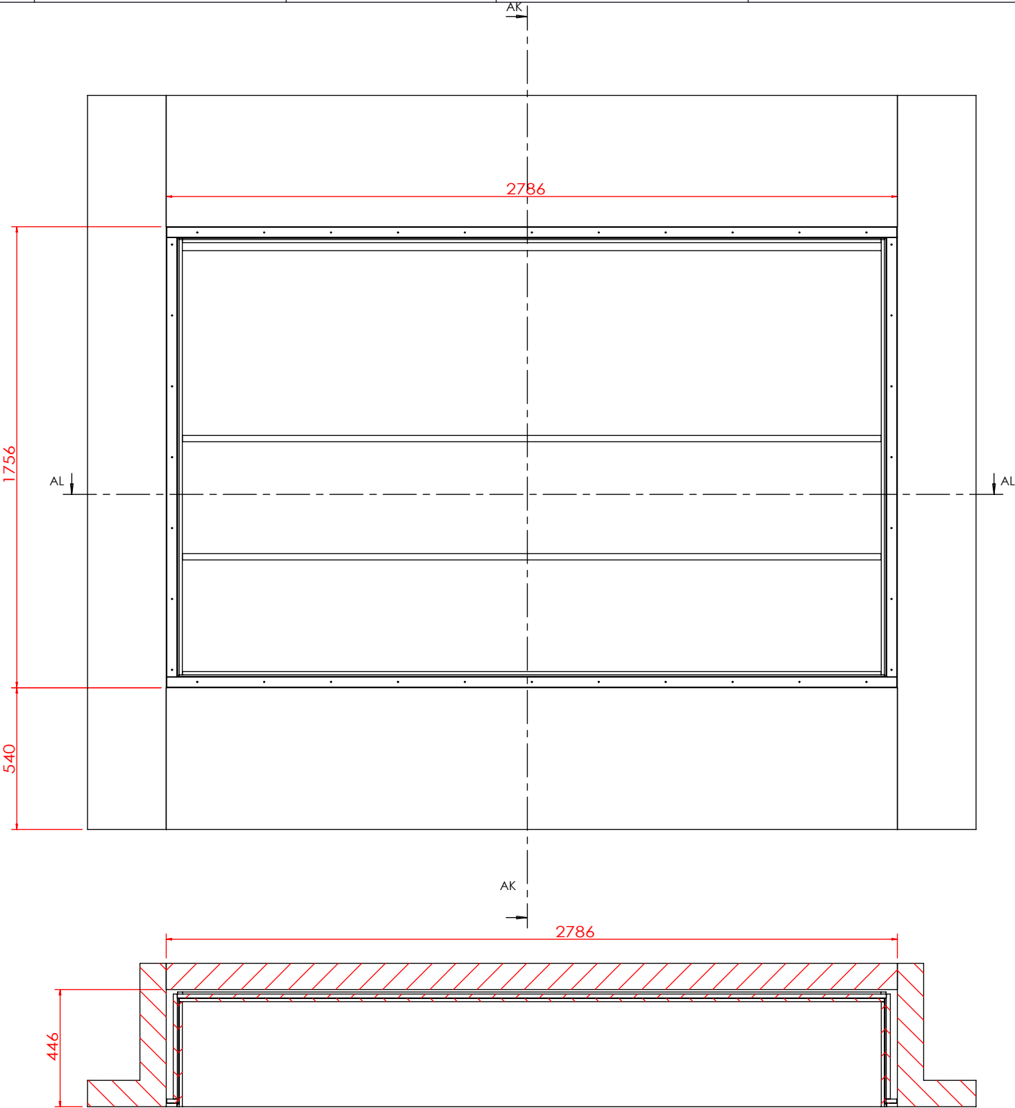
剖面 AL-AL
