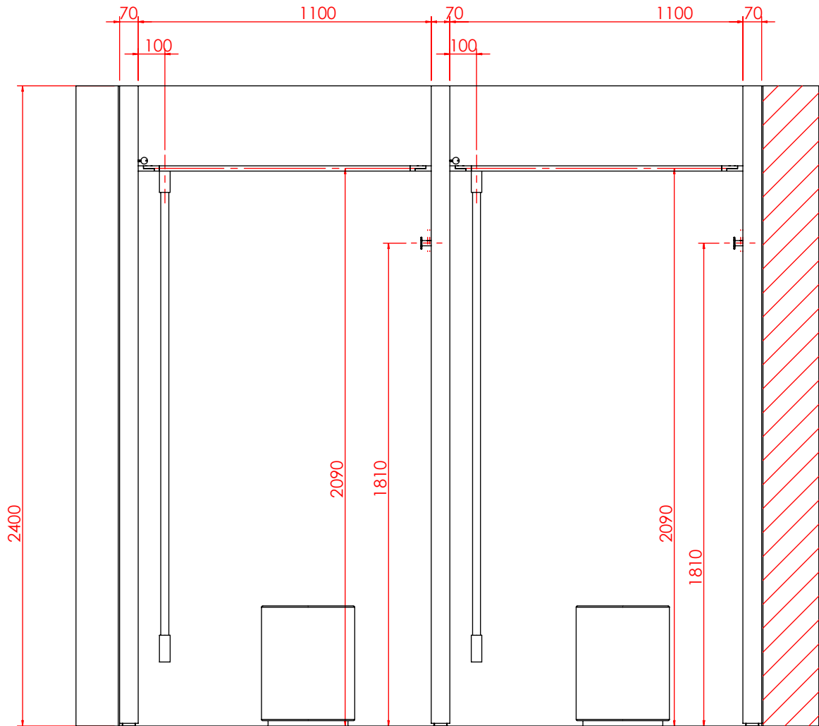
剖面 AG-AG 比例 1 : 20
