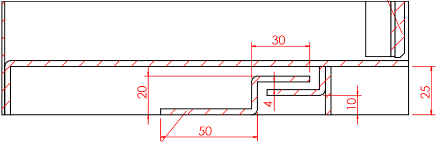
局部视图 AJ 比例 1 : 2
