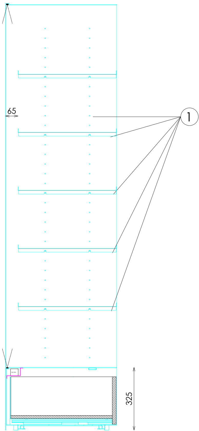
SECCION BALDAS
