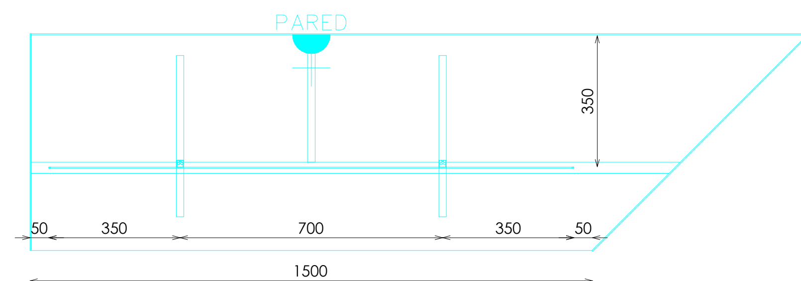
PLANTA BARRA
