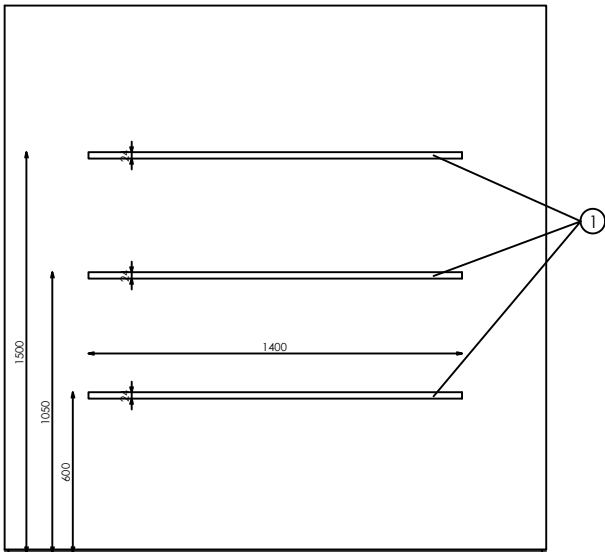
ALZADO
