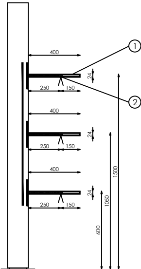
SECCION
