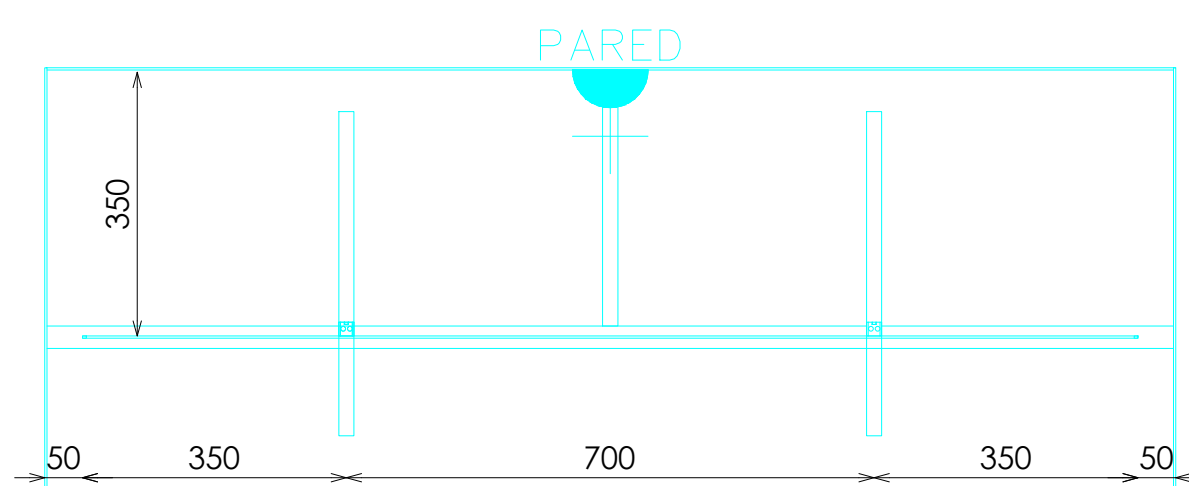
PLANTA BARRA
